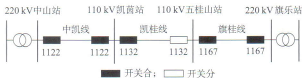
图3 故障前电网结构
